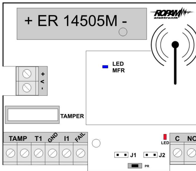
Widok modułu IO-Aero
